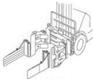
Stipaljka sve u jednom Celuloza / Papir Klizno izmenljivi na ruci.
